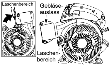
Ansaugöffnungabdeckung
