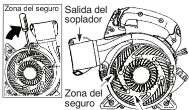
Cubierta de admisión de aspirador
