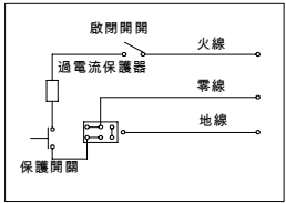
接線圖原理
