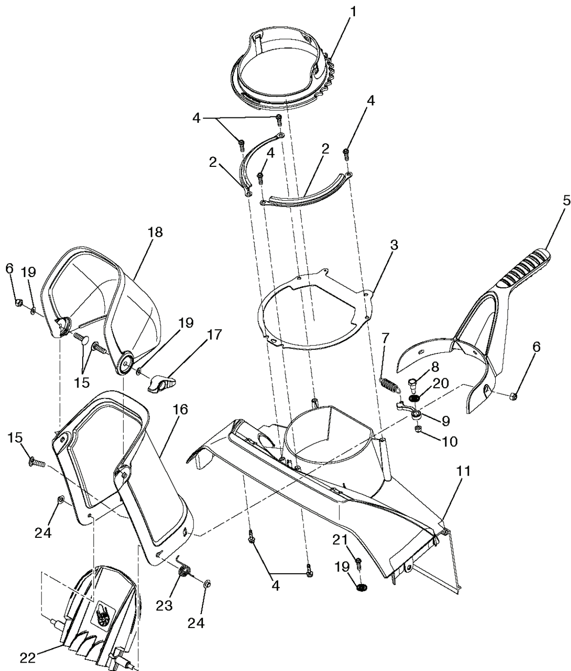
SSST-Chute asm_6
