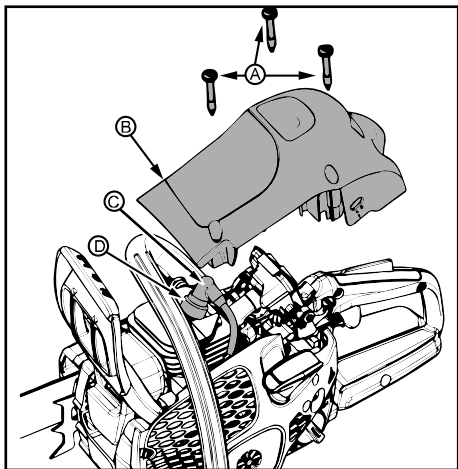
РЕГУЛЮВАННЯ КАРБЮРАТОРА
