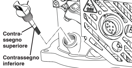
Tappo di rifornimento dell'olio/asta di livello
