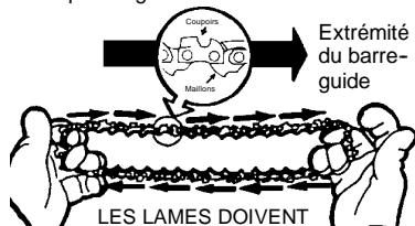
LES LAMES DOIVENT FAIRE FACE DANS LA DIRECTION DE LA ROTATION
