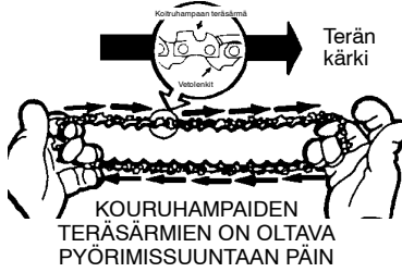
Kouruhampaan teräsärmä Säätöhammas Vetolenkit
