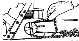
Aseta ketju ketjupyörään
