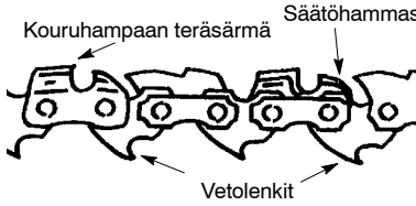
KOURUHAMPAIDEN TERÄSÄRMIEEN ON OLTAVA PYÖRIMISSUUNTAAN PÄIN
