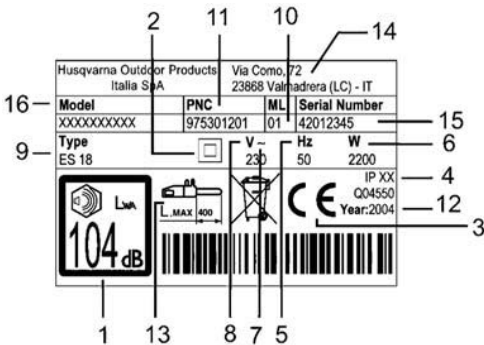
Beispiel für Kennschild
